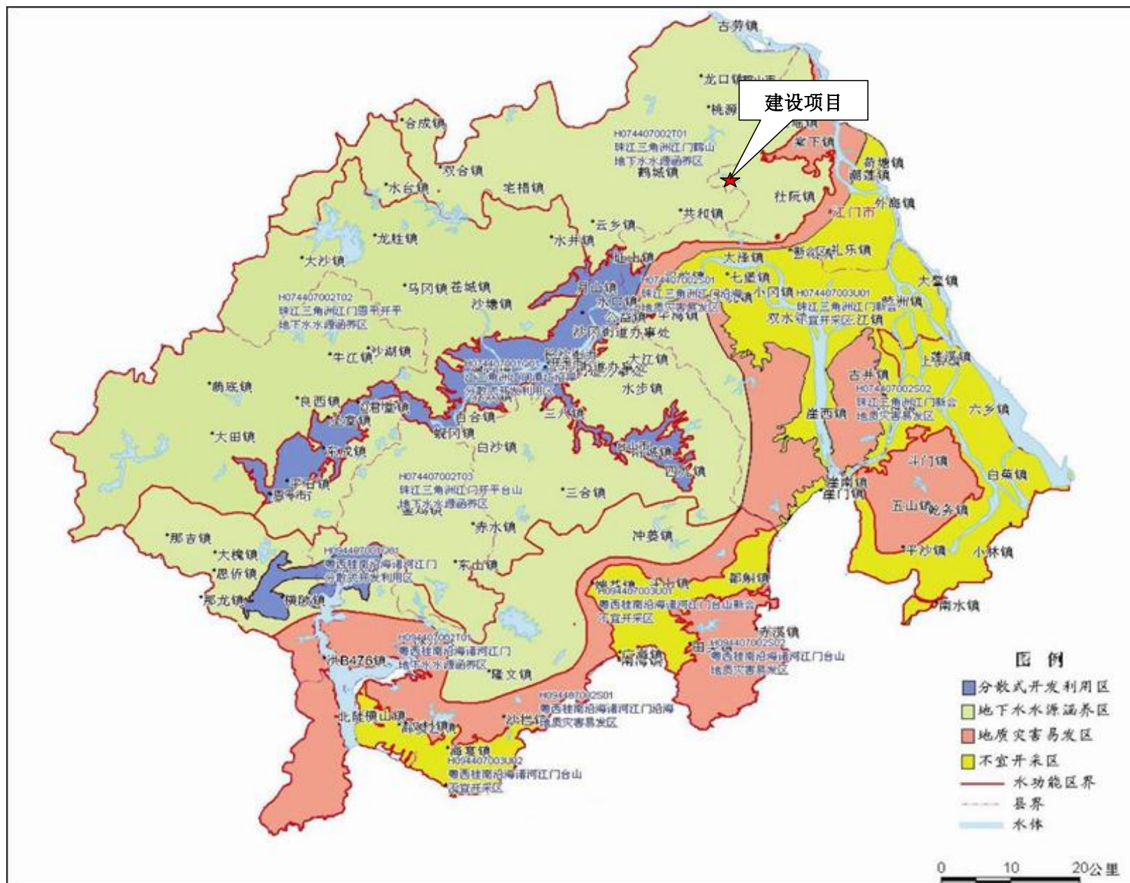
附图 4 江门市地下水功能区划图
