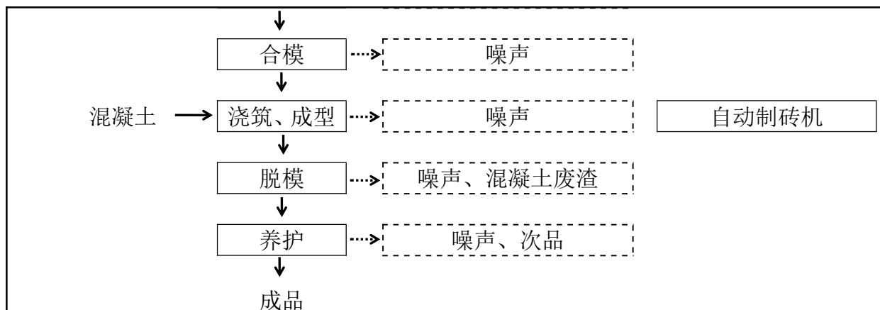
图 2-2 项目生产工艺流程及产排污节点图（路沿石需要脱模剂）
