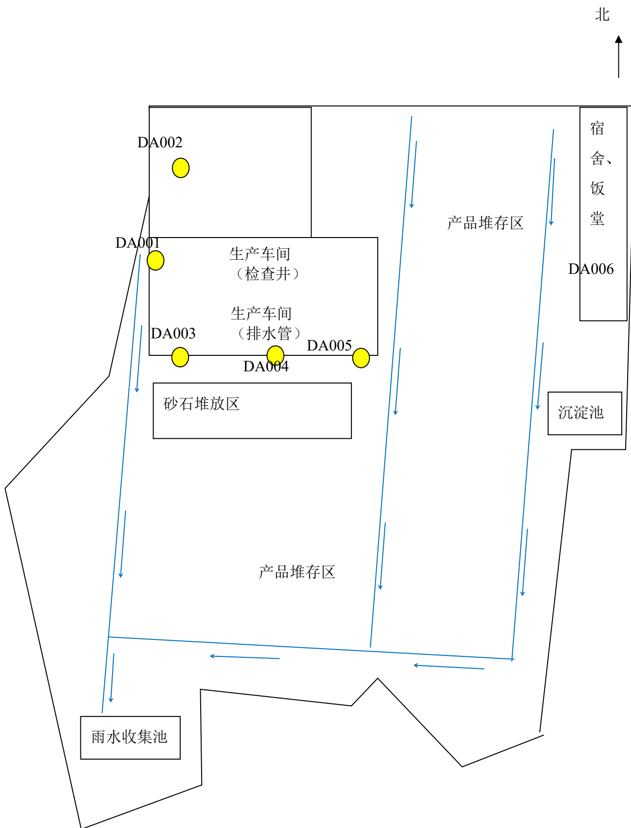
附图 3 雨水管网及流向图
