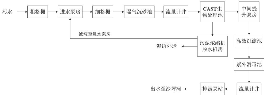
图4-2 鹤山市第二污水处理厂采取的处理工艺流程图
