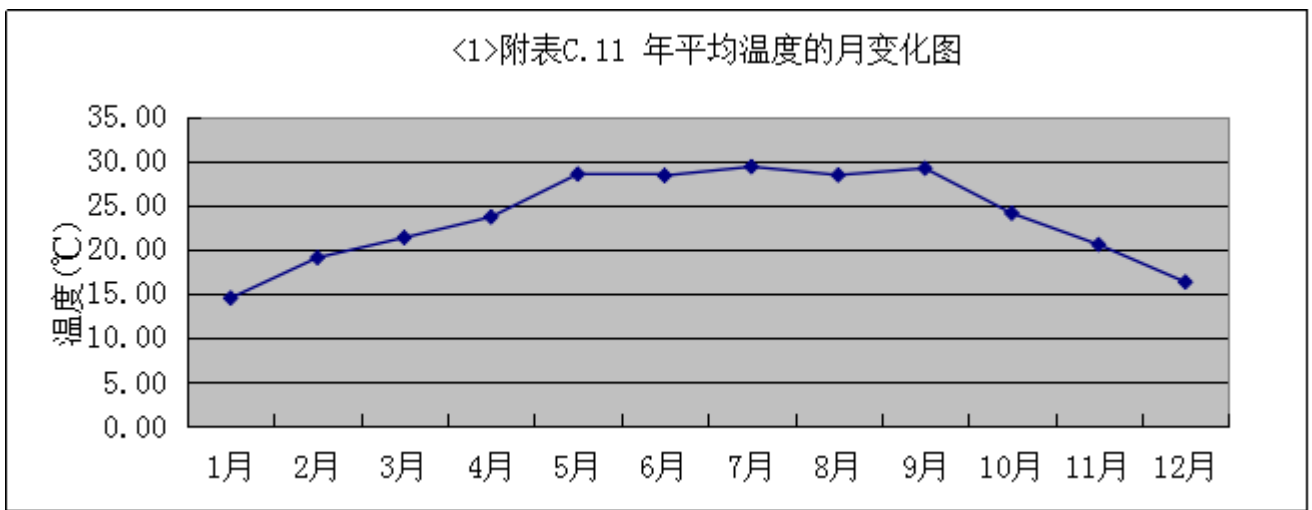
图 6.2-12 项目所在区域 2021 年平均温度月变化图
