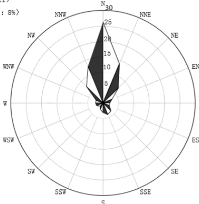
图 6.1-2 鹤山 20 年累年月风向玫瑰图
