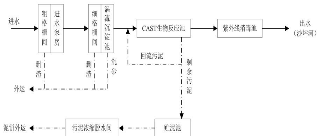
图 4-1 鹤山市第二污水厂工艺流程图
